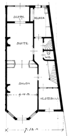
AFB.211 Doornstraat 9, begane grond, plattegrond aangepast aan het perceel, HJD, 9 juni 1903
